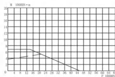
图 4 WD-23.20.0744
