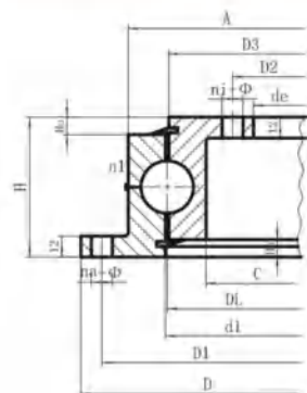
WD-230
