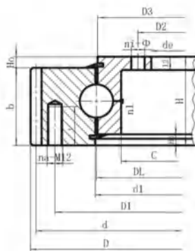
WD-231
