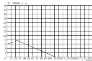
图 3 WD-06.20.0644
