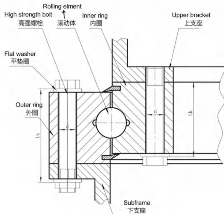
安装示意图 Installation schematic
