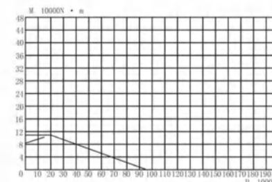
图 2 WD-06.20.0544
