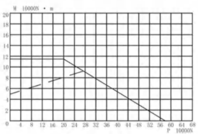
图 3 WD-23.20.0944
