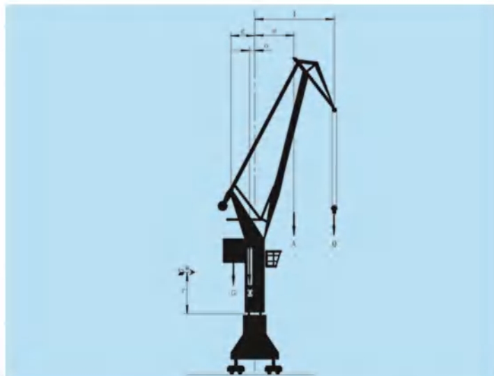
门座式起重机示意图 The portal crane diagram
