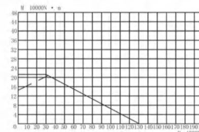
图 4 WD-06.20.0744
