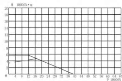
图 3 WD-23.20.0644
